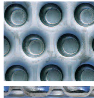
Комбинированная перфорация
