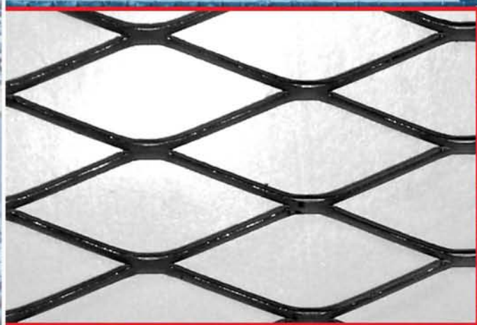
Просечно-вытяжной лист TR 62 x 21 x 2,5 x 2 мм
