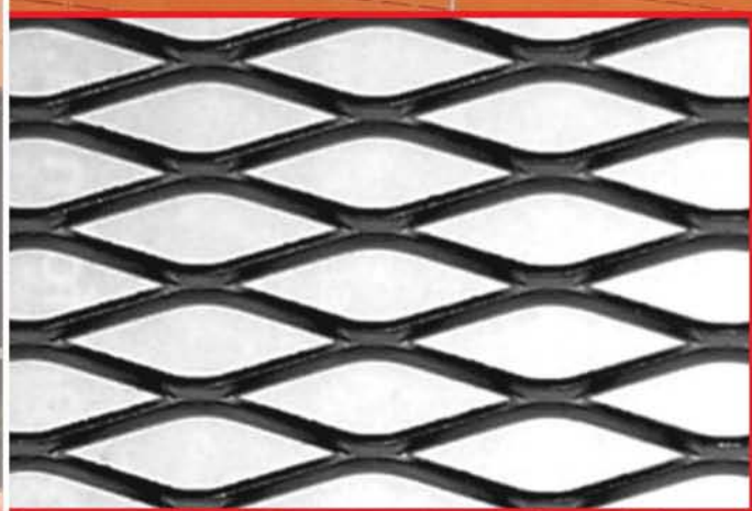
Просечно-вытяжной лист TR 42 x 13 x 2,5 x 1,5 мм
