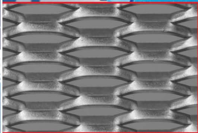
Просечно-вытяжной лист ТН 47 x 13 x 4 x 2 мм
